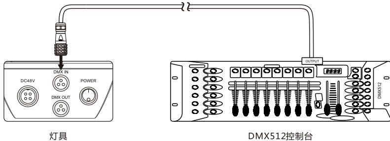
DMX-单灯连接图
