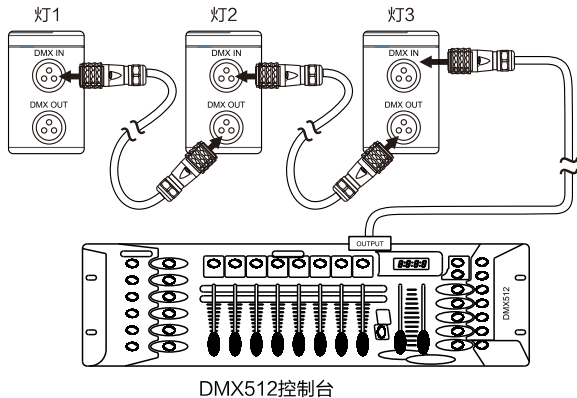
DMX-多灯连接图
