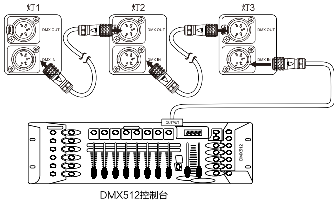
DMX-多灯连接图
